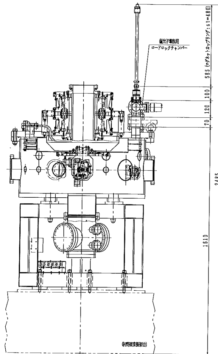
Y-Y断面図
